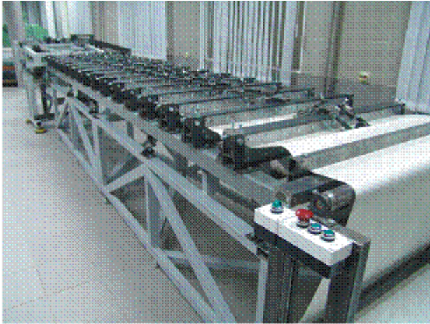
Установка для циклического формования z-гофра из бумаги Nomex
