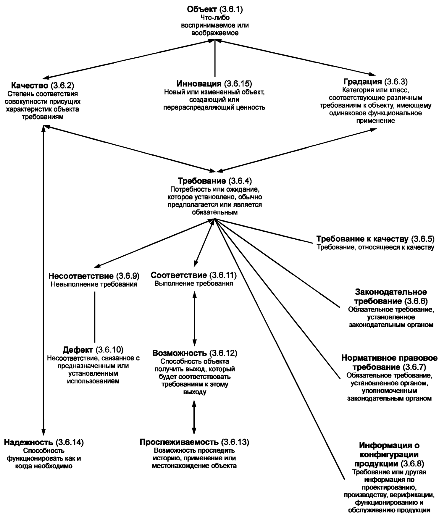
Рисунок А.9 — 3.6 Понятия, относящиеся к категории «требование»
